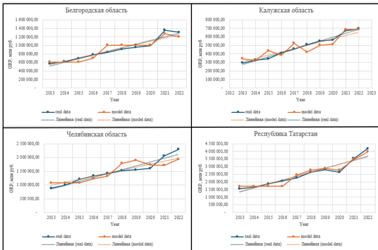
Рис. 2. Графики реальных и моделируемых данных. Данные рассчитаны и получены автором в MS Excel
